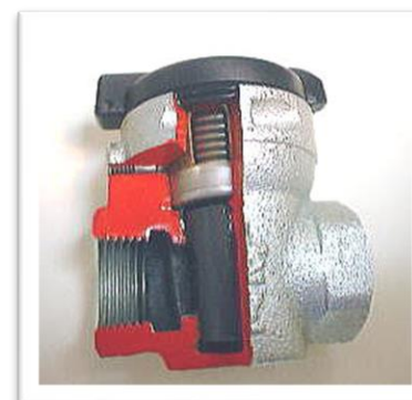
感熱自動閉止ガス栓
